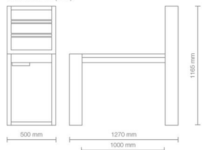
DIMENSIONI (mm)
